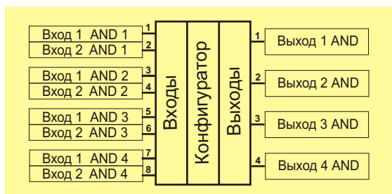
Рис. 58. Блок “Логическое И”, тип “2 AND”
