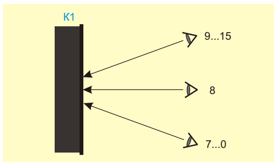
Рис. 21. Оптимальные значения задатчика яркости в зависимости от угла обзора (только для экранов с ЖКИ-дисплеем)
