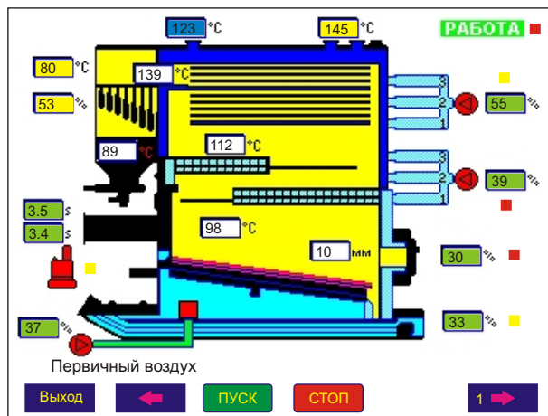
Рис. 153. Меню "Процесс" (Блок "SCADA"). Пример отображения работы твердотопливного котла.
