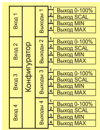
Рис. 24. Выходы функционального блока Аналоговый ввод
