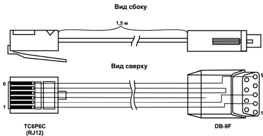
Рисунок Д.1 – Схема кабеля KC1
