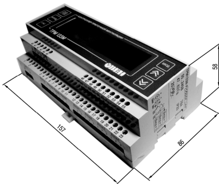
Рисунок А.1 – Корпус для крепления на DIN-рейку 35 мм
