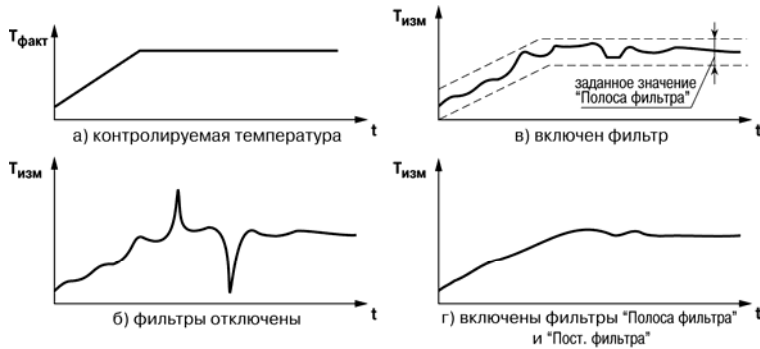
Рисунок 3.3 – Временные диаграммы работы цифровых фильтров показаний датчика
