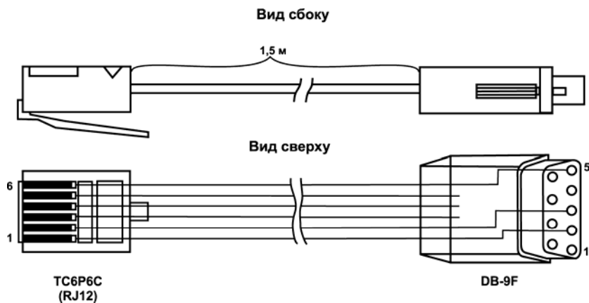
Рисунок Д.2 – Схема кабеля KC2
